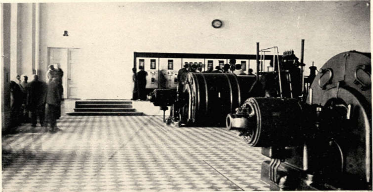
Turbogeneraatorid Ulila elektriijaamas.
