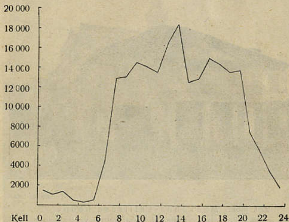
221. joon. Jalakäijate liikimise kõver
