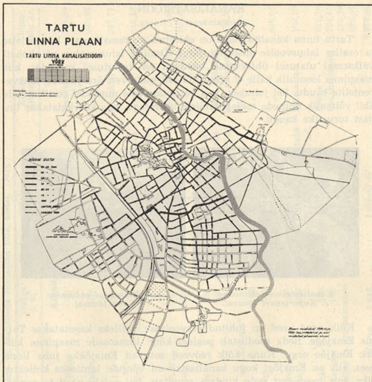
Tartu linna kanalisatsioonivõrk.
